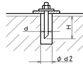
アンカーボルト施工図
