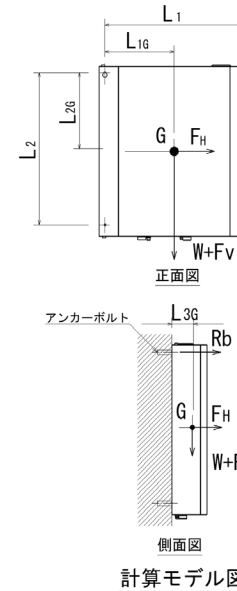
計算モデル図
