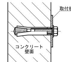
アンカーボルト施工図
