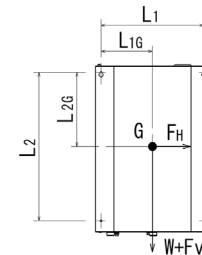
正面図
