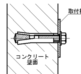
アンカーボルト施工図
