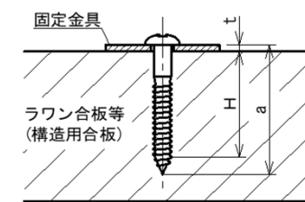
アンカーボルト施工図
