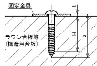
アンカーボルト施工図
