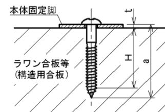
(十字穴付き丸木ねじ)
