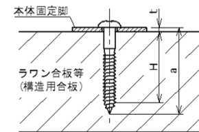
アンカーボルト施工図
