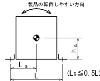
計算モデル図
