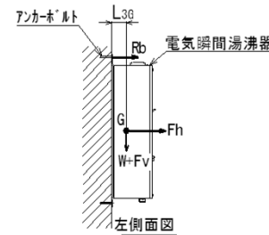
左側面図 計算モデル図
