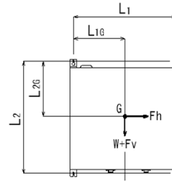
背面図 (後側から見た図)
