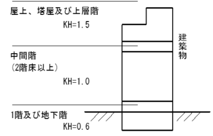
局所震度法による設計用震度 (通常の建築設備 地域係数=1)
