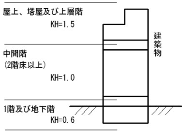
局所震度法による設計用震度 (通常の建築設備 地域係数=1)
