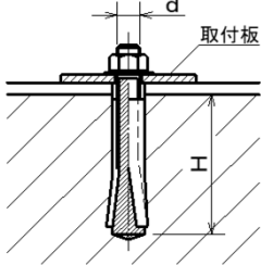
アンカーボルト施工図
