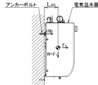
左側面図 計算モデル図
