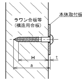
アンカーボルト施工図 (十字穴付き丸木ねじ)
