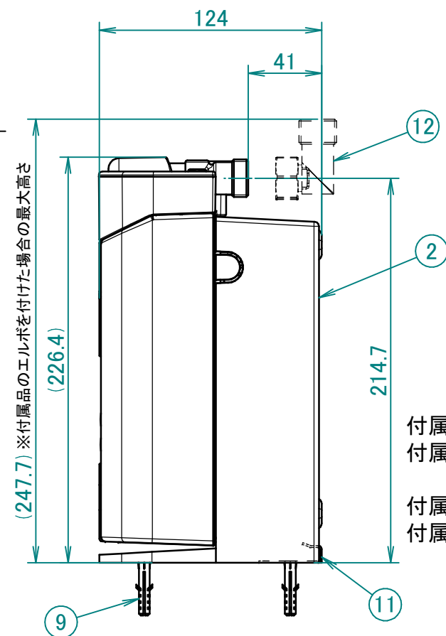
右側面図
