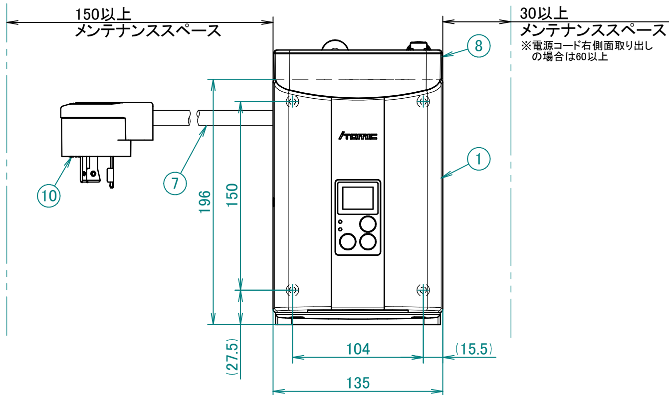
正面図
