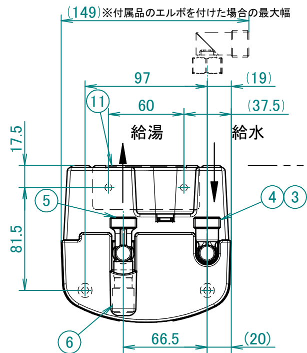
上面図
