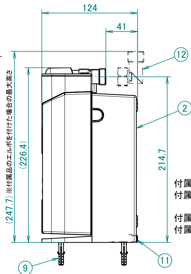
右側面図
