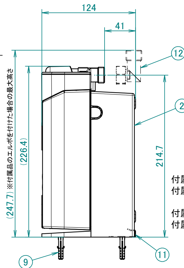
右側面図
