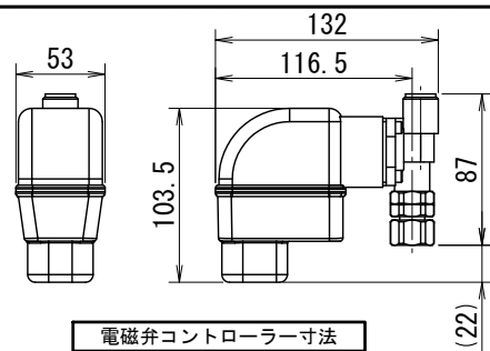
電磁弁コントローラー寸法
