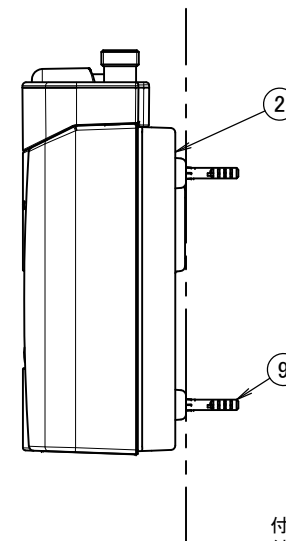
右側面図
