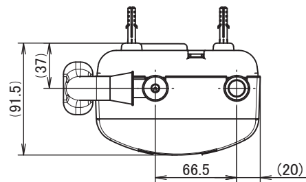
上面図
