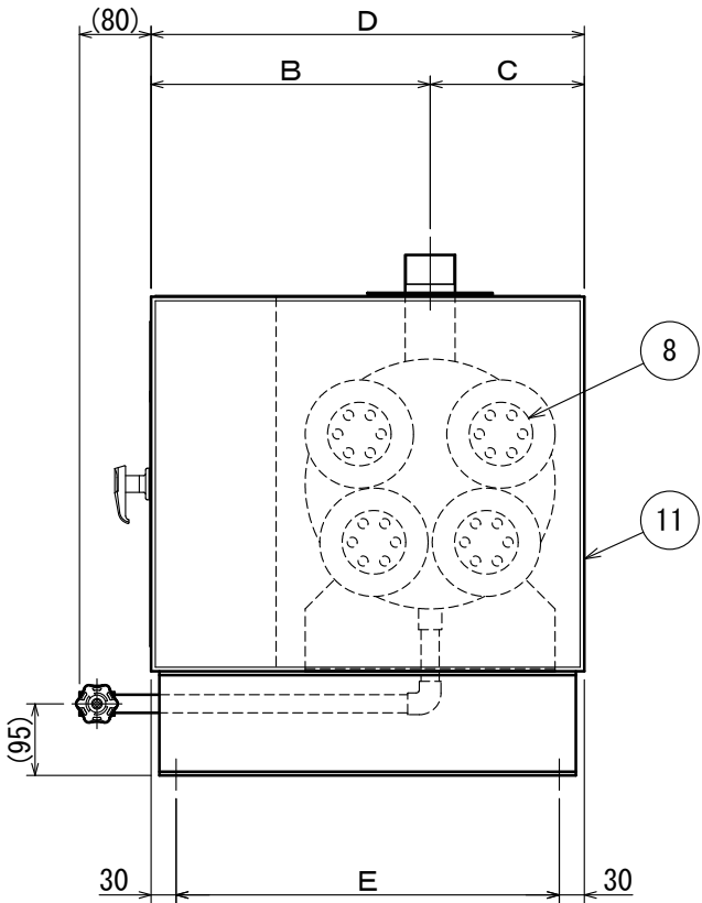
右側面図
