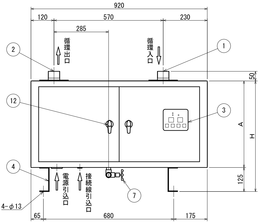
正面図
