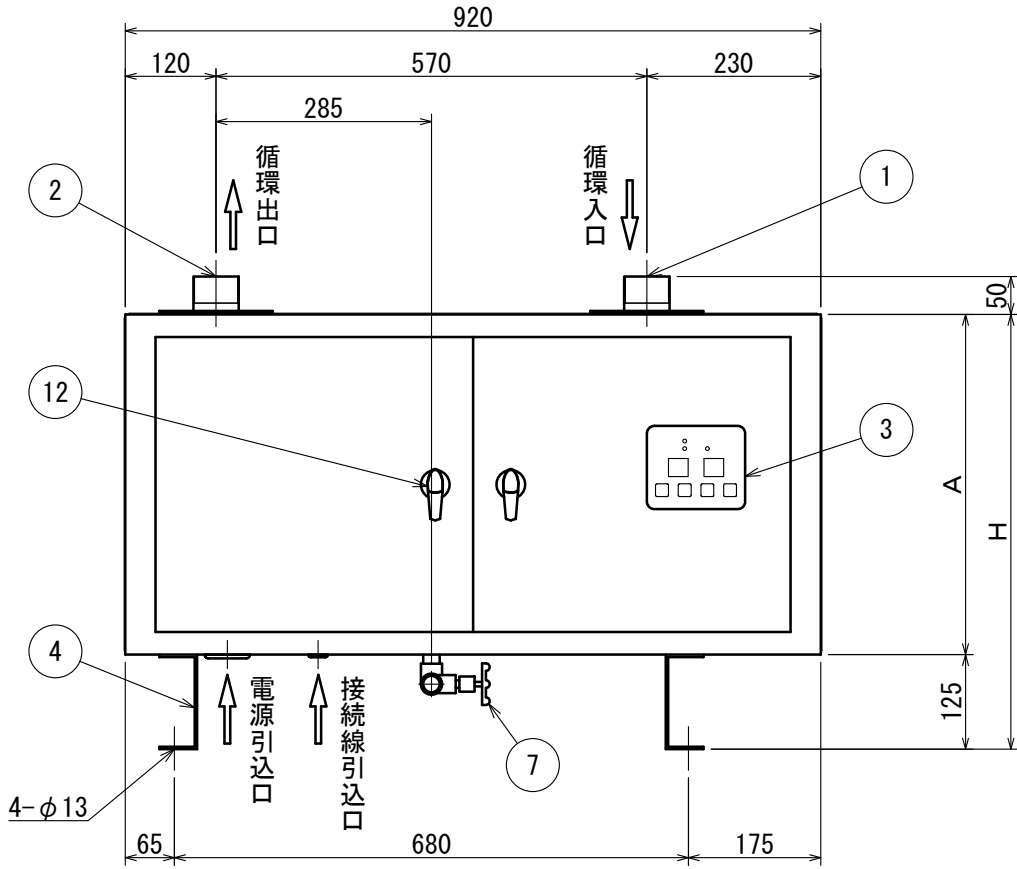
正面図
