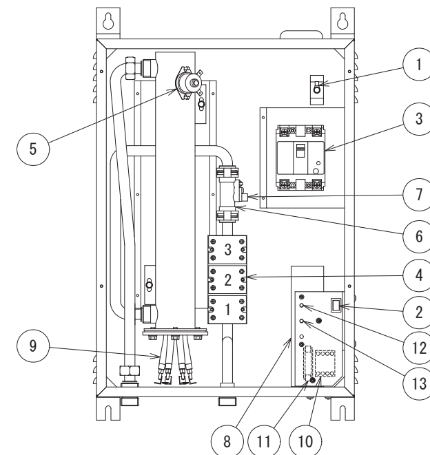
部品配置図
