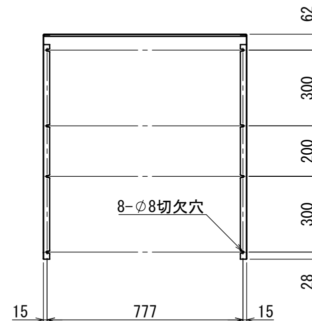
断面図 B-B
