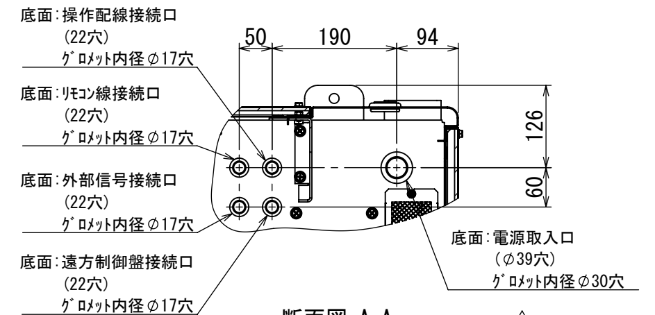
断面图 A-A
