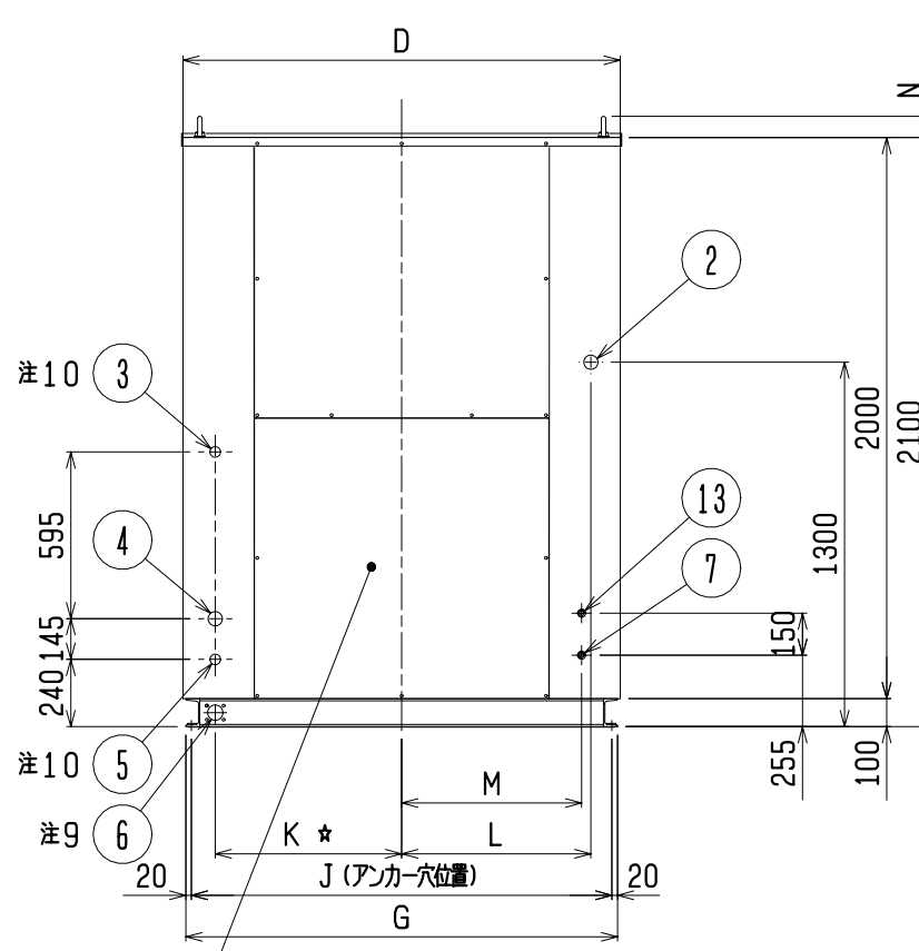
右側面図
