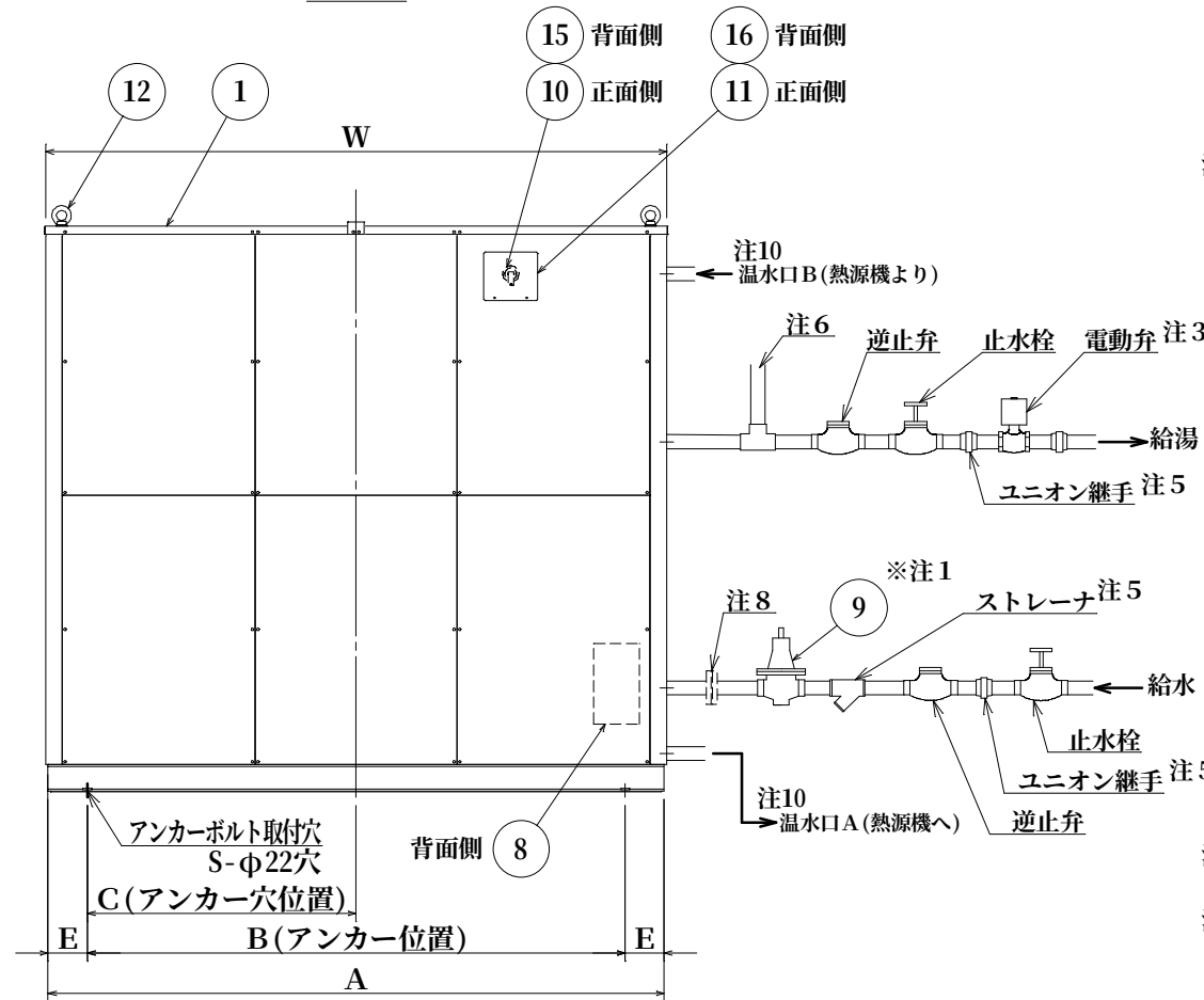
正面図
