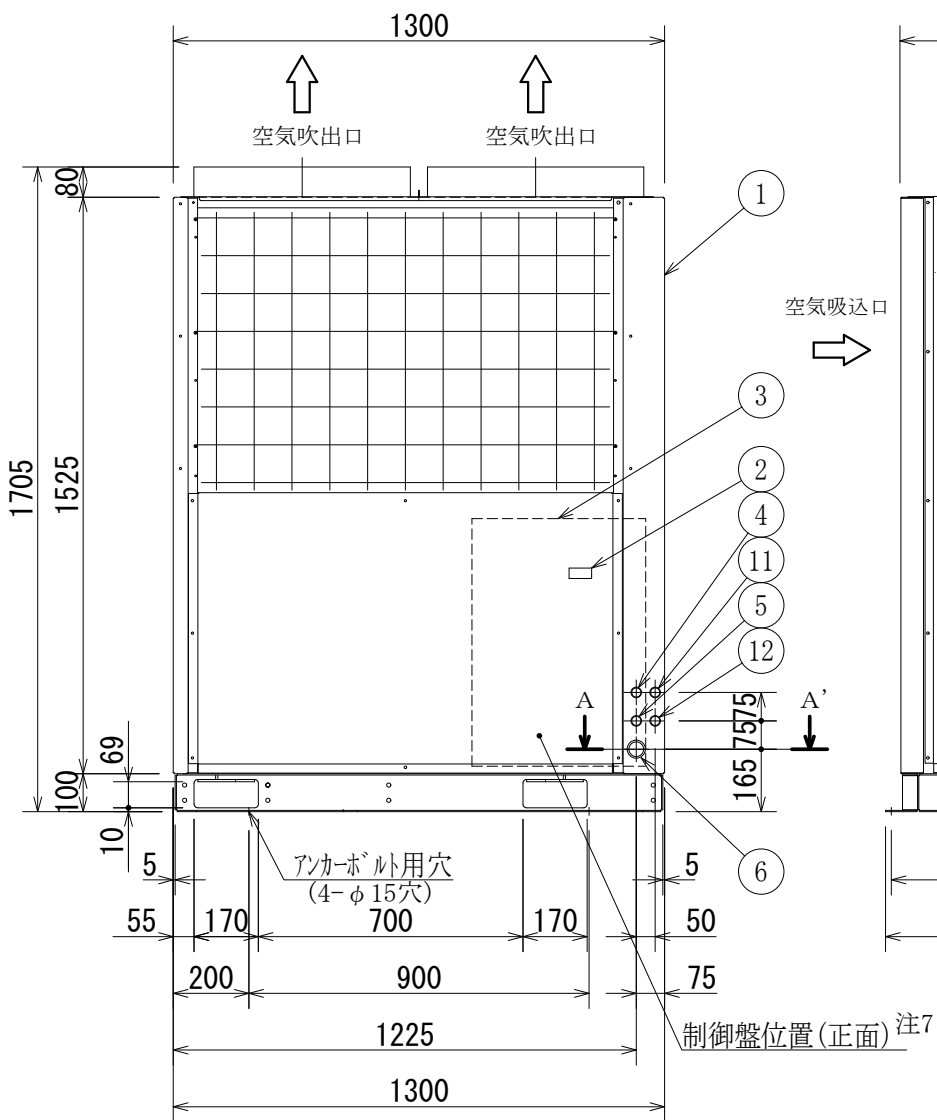
正面図
