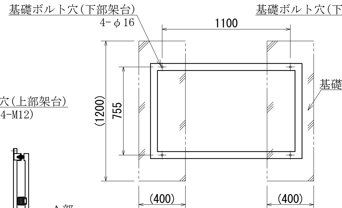
基礎 寸法図
