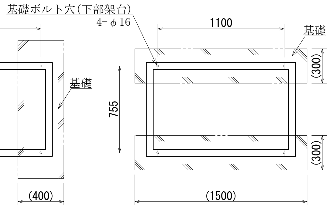
基礎 寸法図
