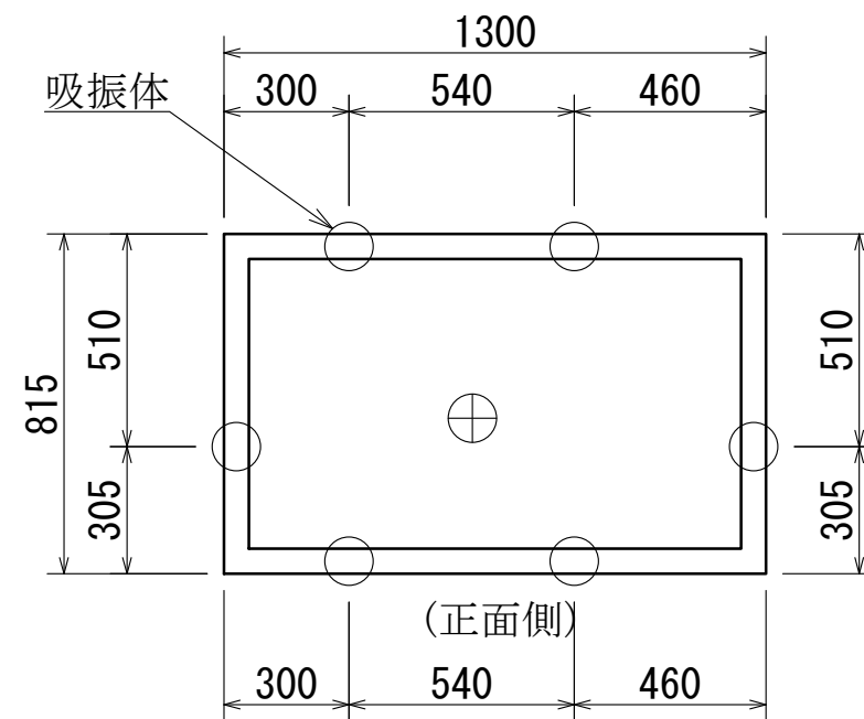
吸振体配置図
