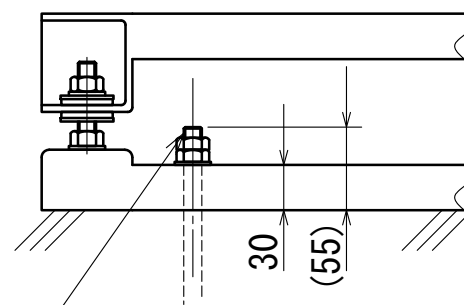
A部詳細図(1:5)
