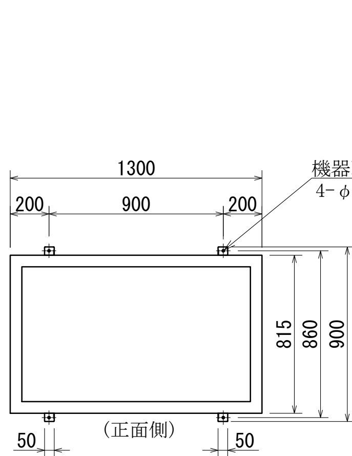
平面図
