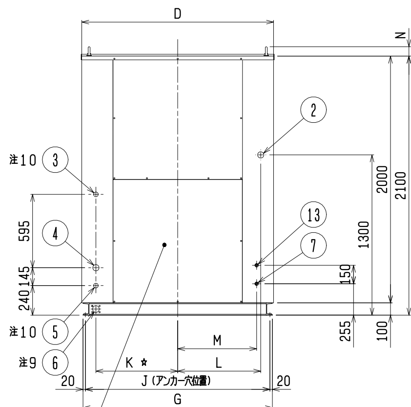
右側面図
