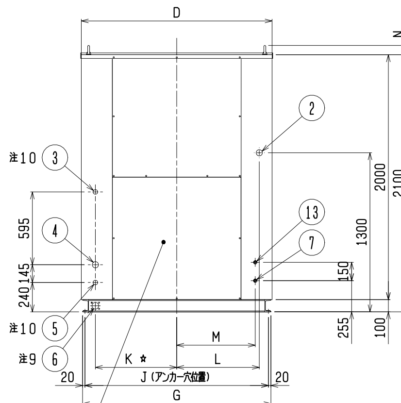
右側面図
