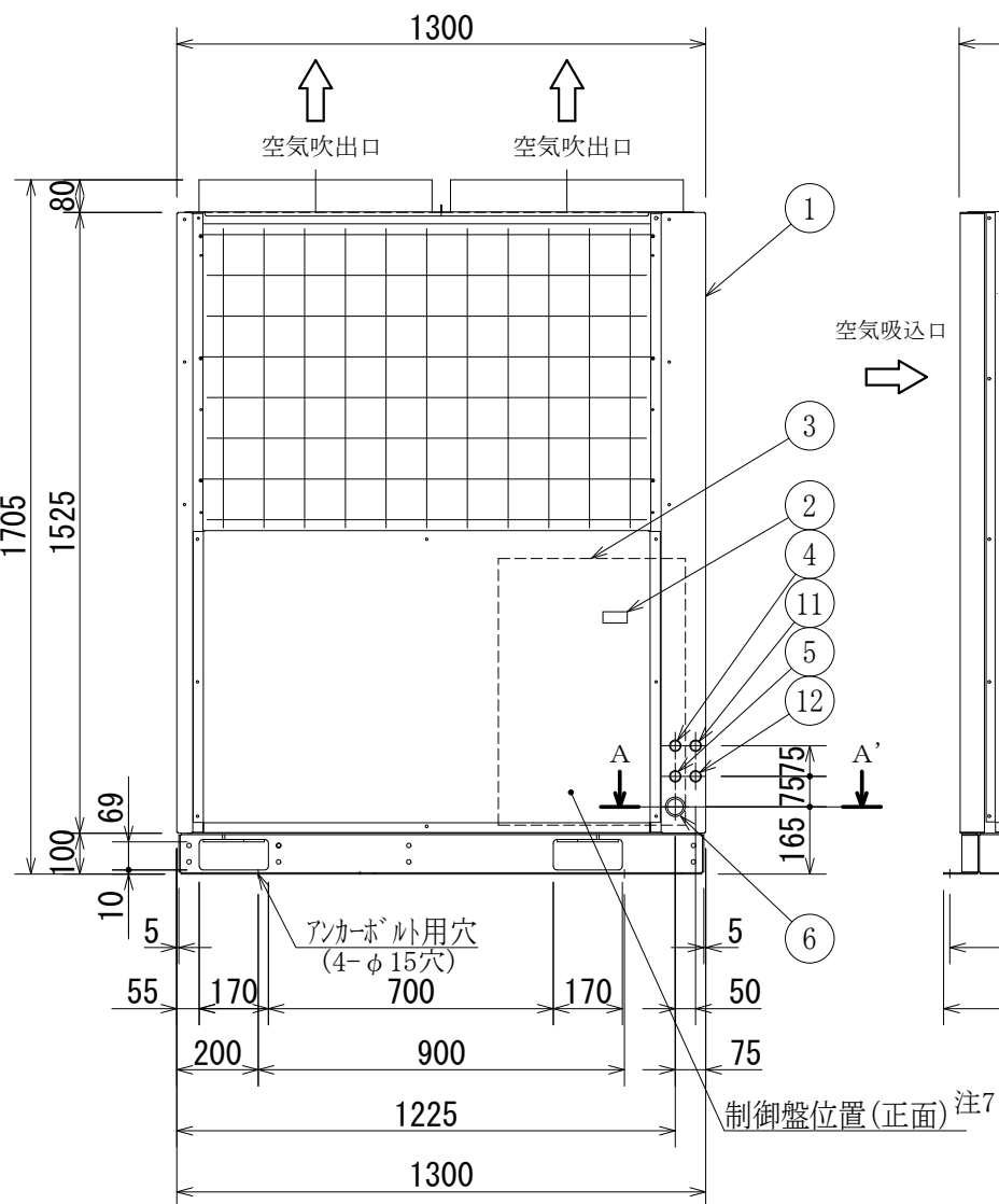
正面図
