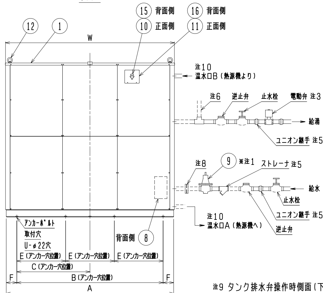
平面図
