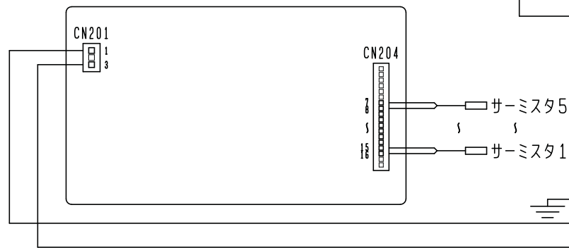
タンクセンサ基板
