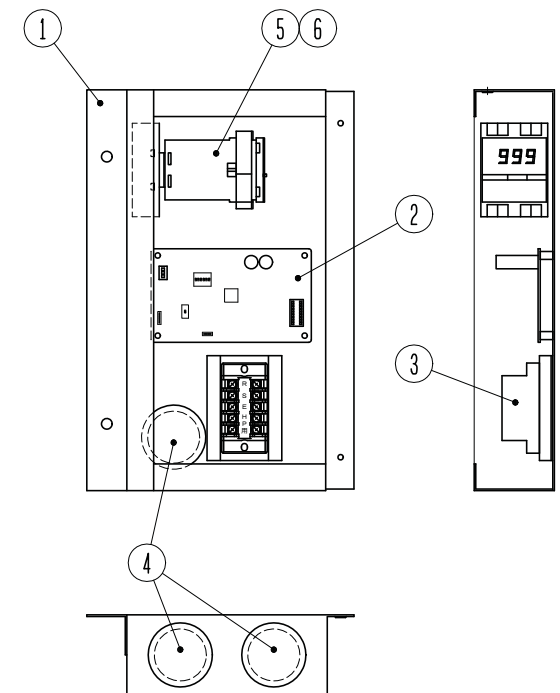
連絡線接続BOX内部品配置図
