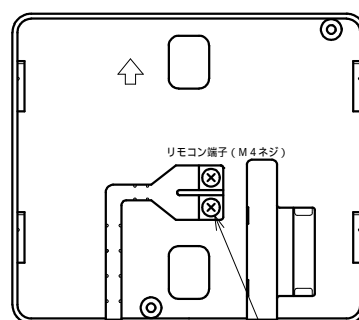
背面図
