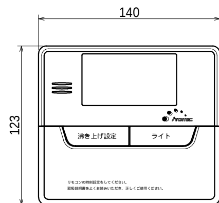
正面図
