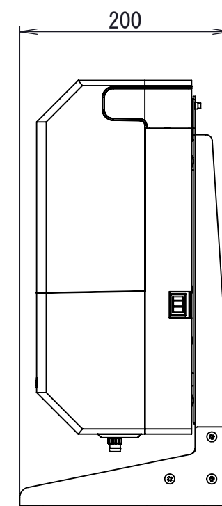
温水器(正面カバー取付状態)組立時寸法
