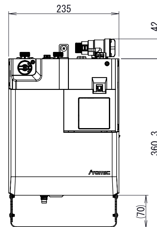
温水器(正面カバー取り外し状態)組立時寸法
