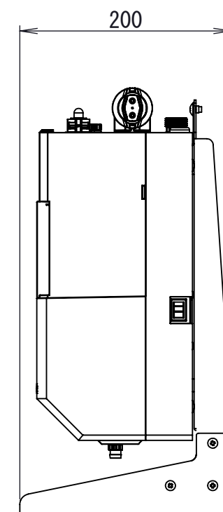
温水器(正面カバー取り外し状態)組立時寸法
