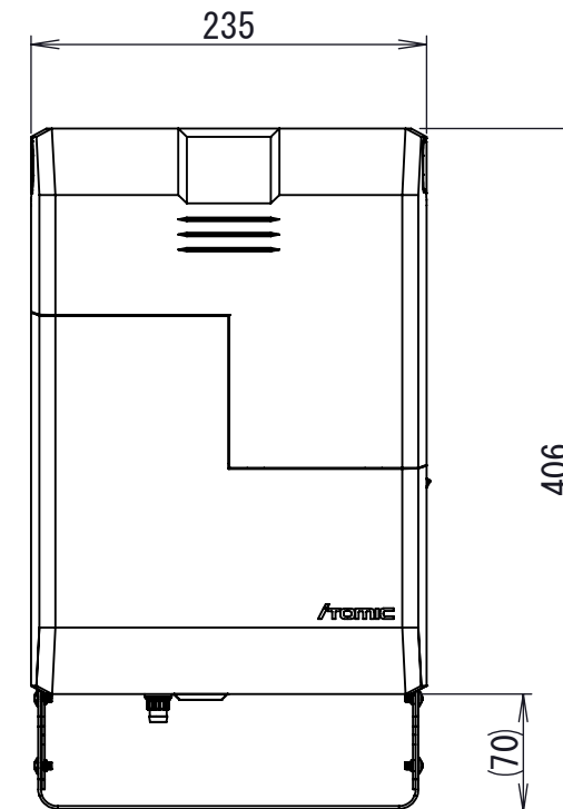
温水器(正面カバー取付状態)組立時寸法
