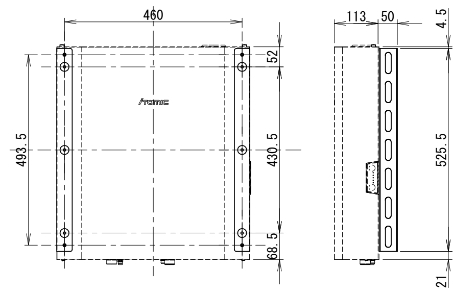
【EIZ-3□00A0(30・40kW)離隔取付金具 取付位置】
