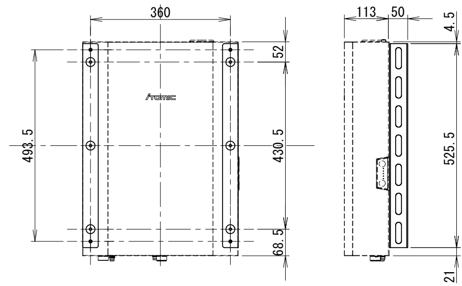
【EIZ-3□00A0(30・40kW)離隔取付金具 取付位置】
