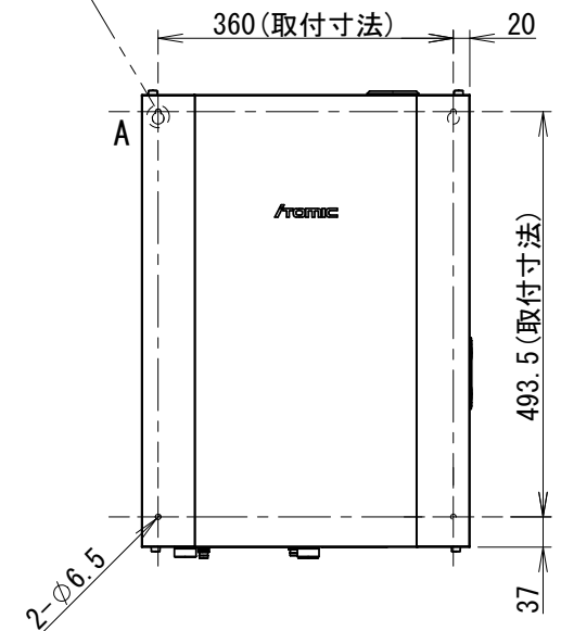
【固定ねじ穴位置図】
