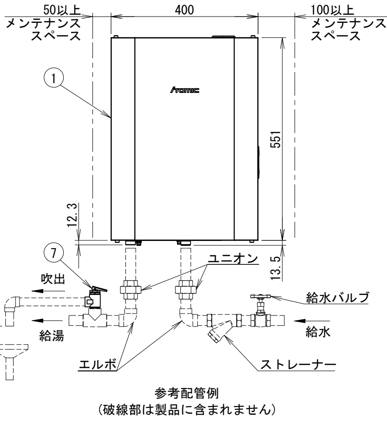
【正面図】
