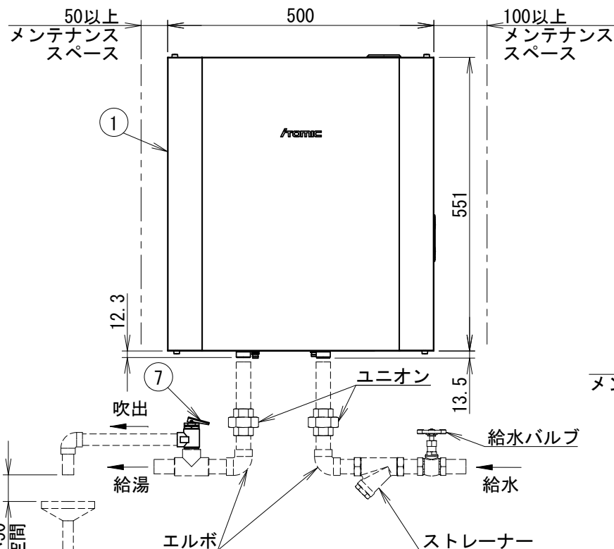
参考配管例 (破線部は製品に含まれません)
