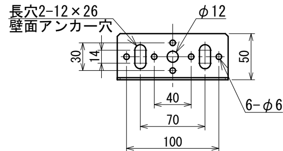
上部固定金具詳細
