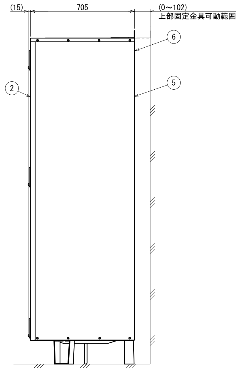
右側面図
