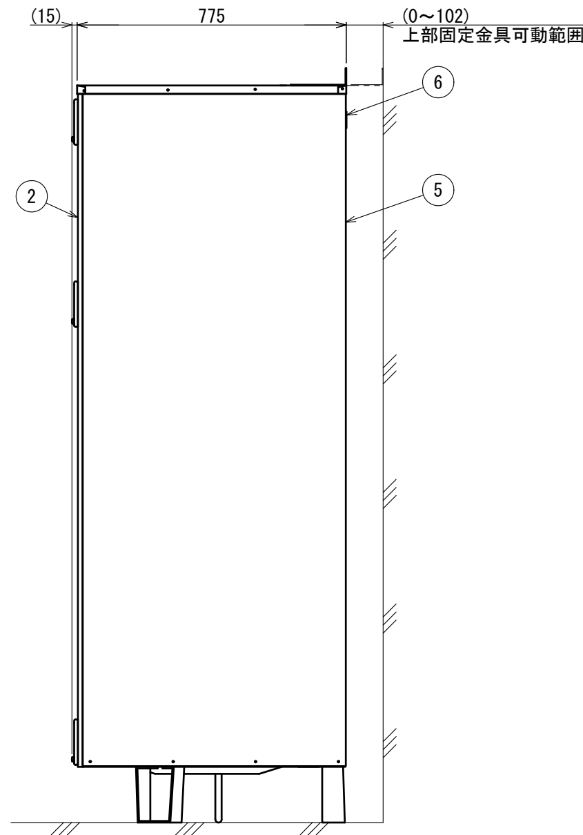
右側面図
