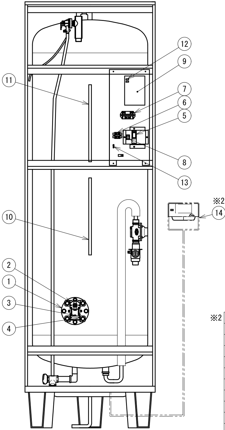
部品配置図
