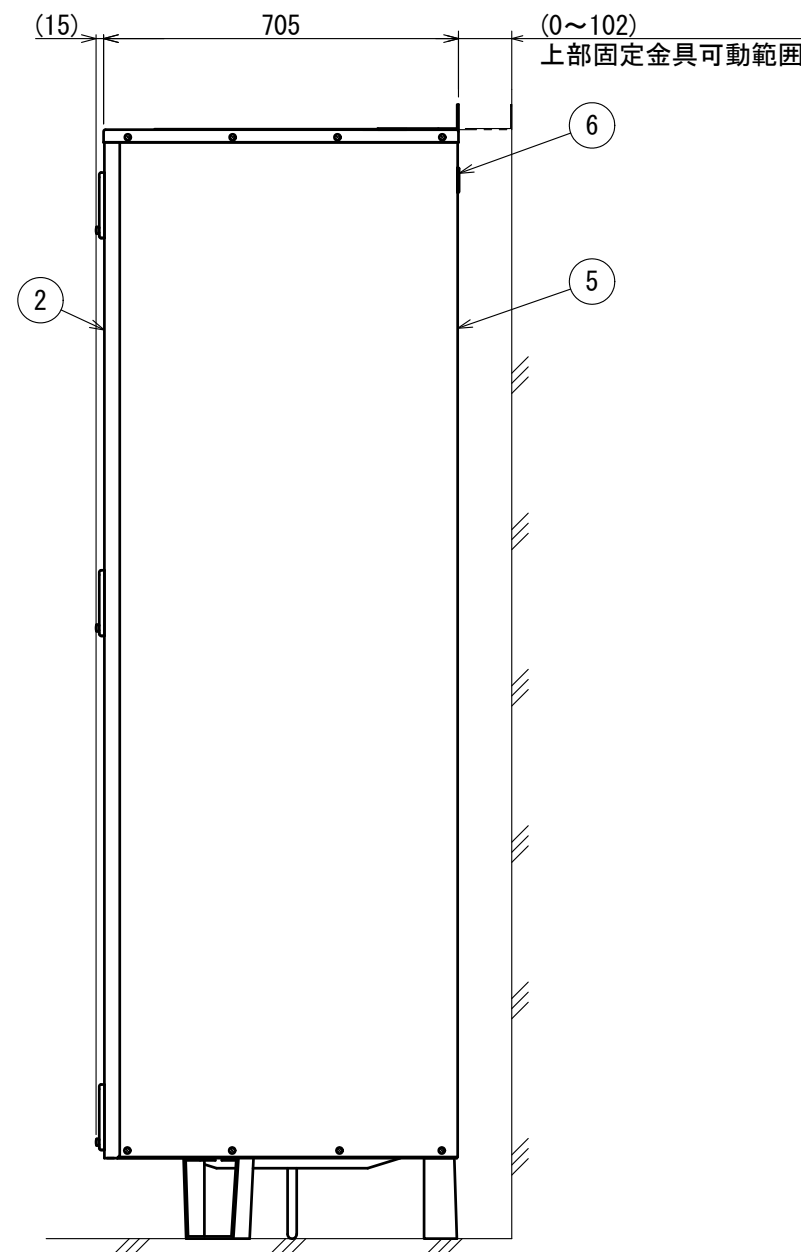
右側面図
