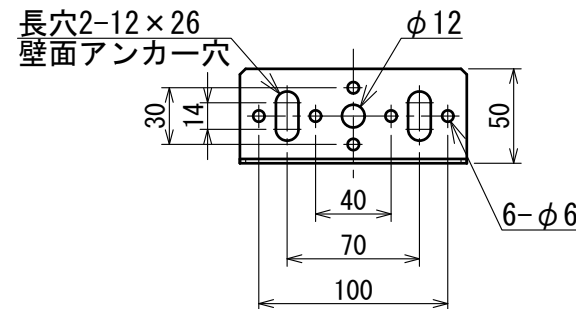
上部固定金具詳細
