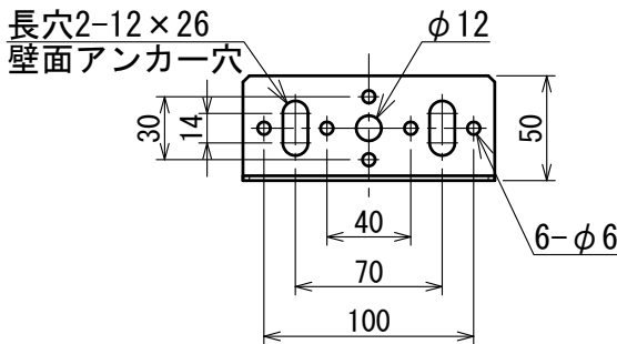
上部固定金具詳細
