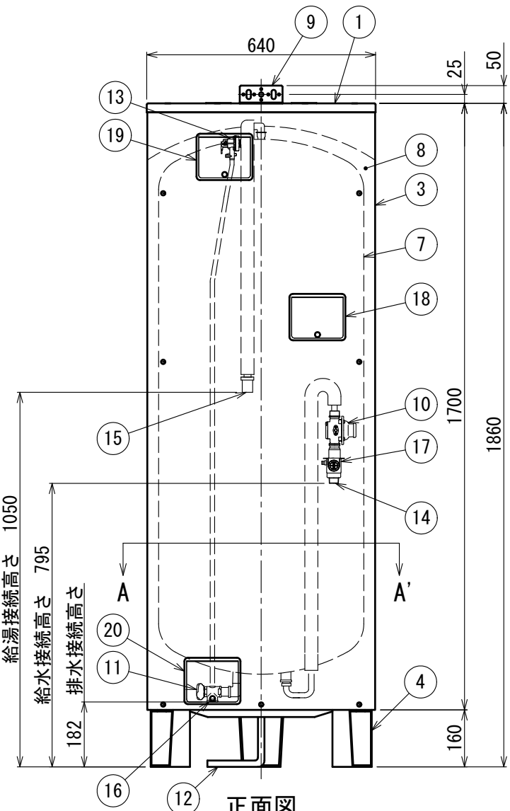
正面図
