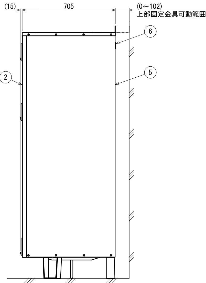
右側面図
