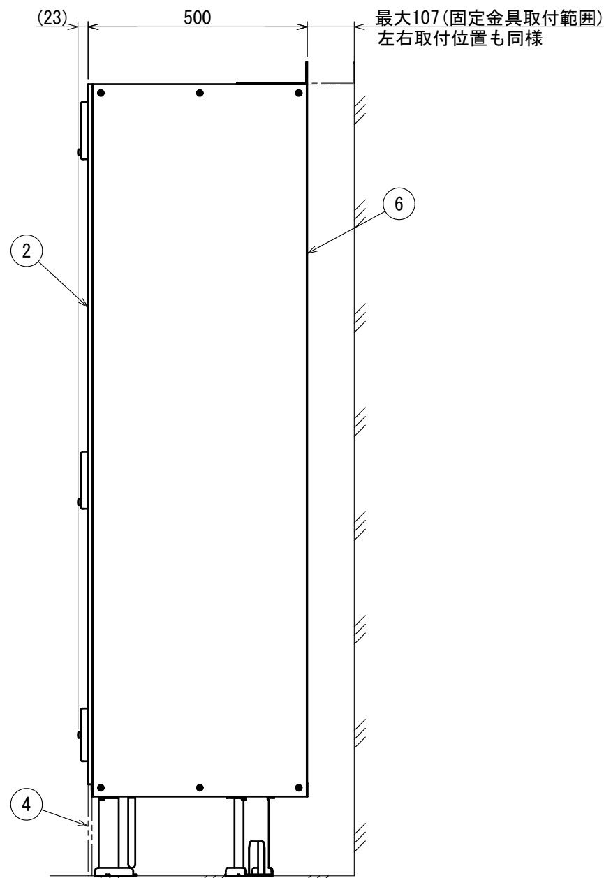
右側面図
