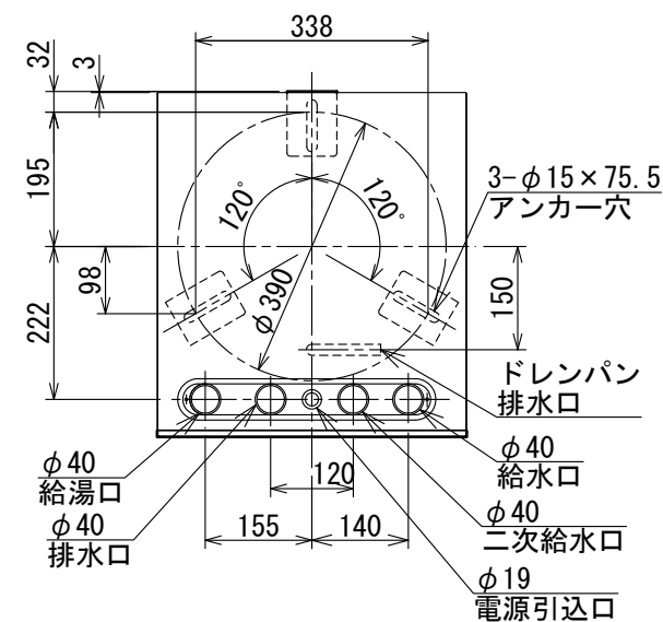
A-A' 断面図(上から見た図)
