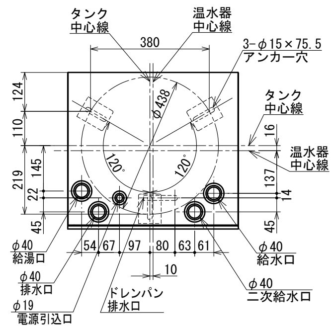
A-A' 断面図(上から見た図)
