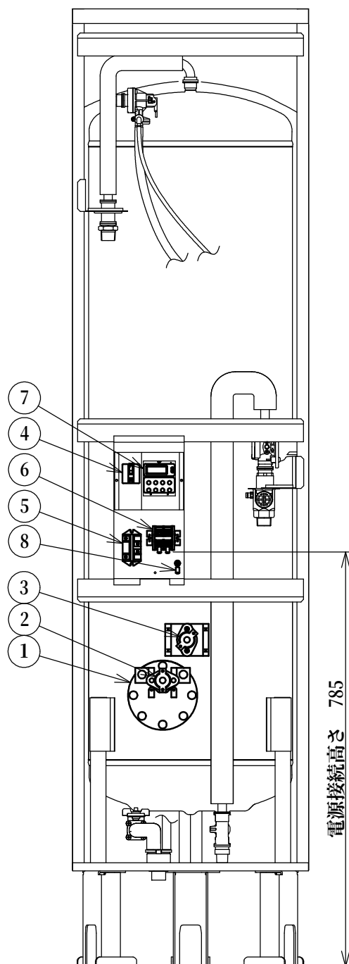
部品配置図 (図はES-150RTS)
