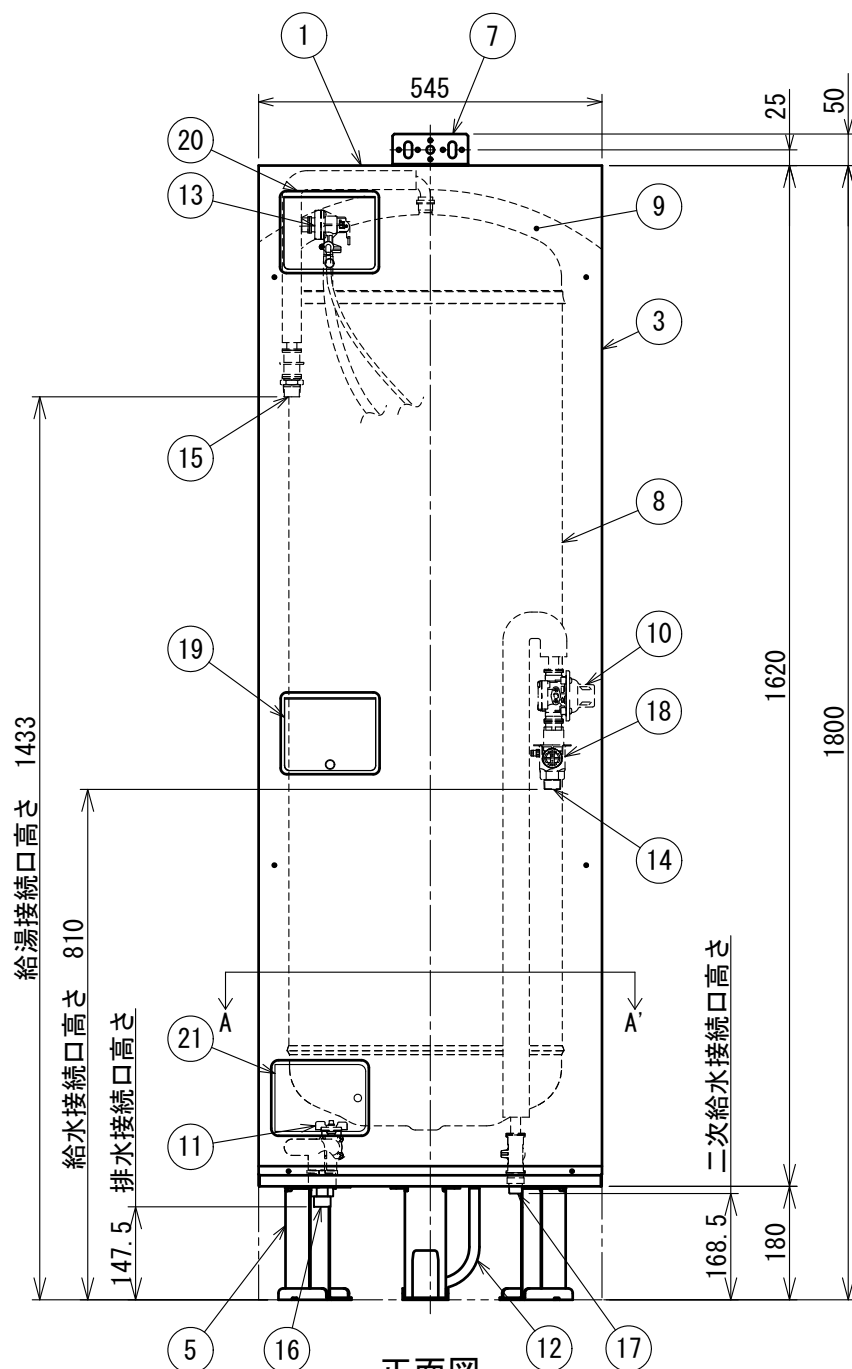
正面図
