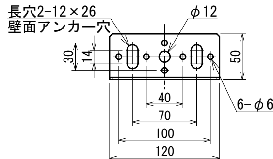
上部固定金具詳細
