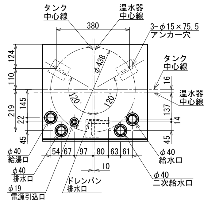
A-A' 断面図(上から見た図)
