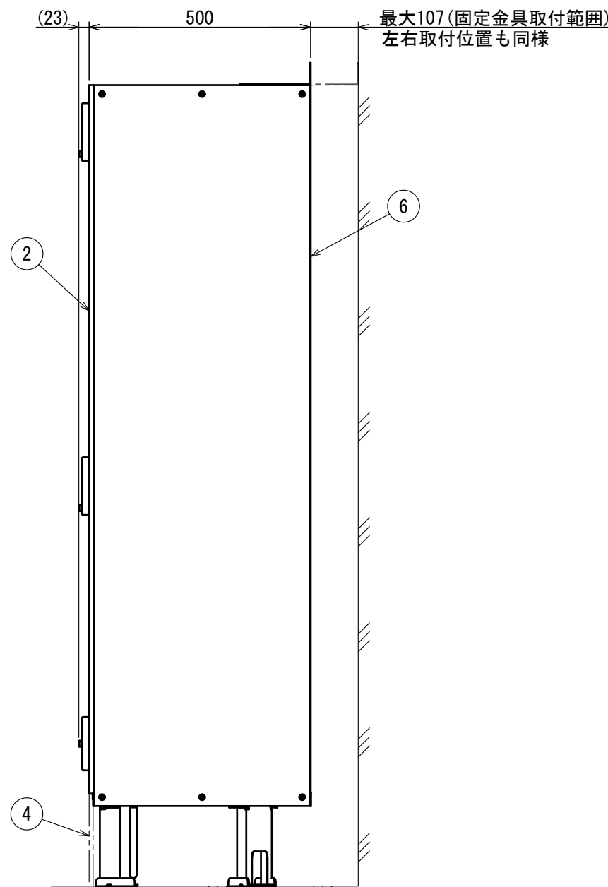
右側面図
