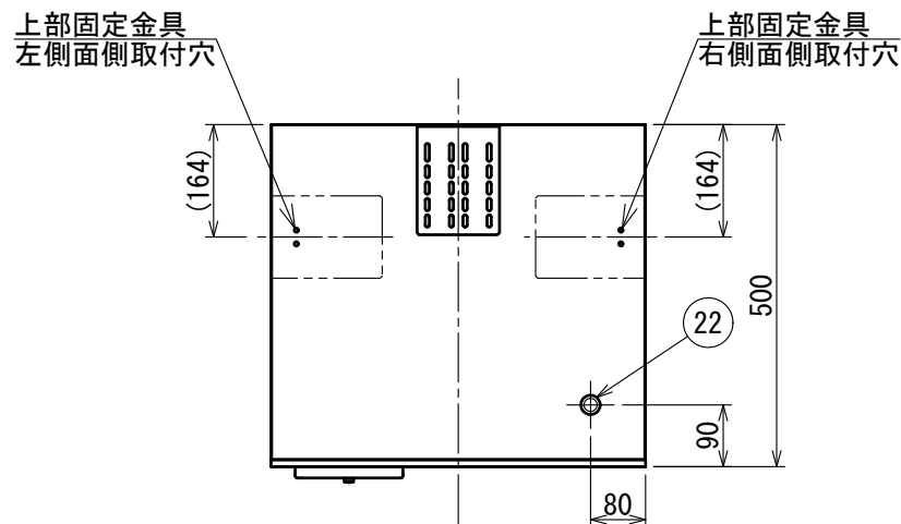
平面図
