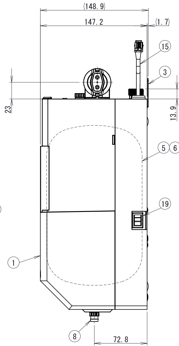
正面カバー取り外し状態詳細図
