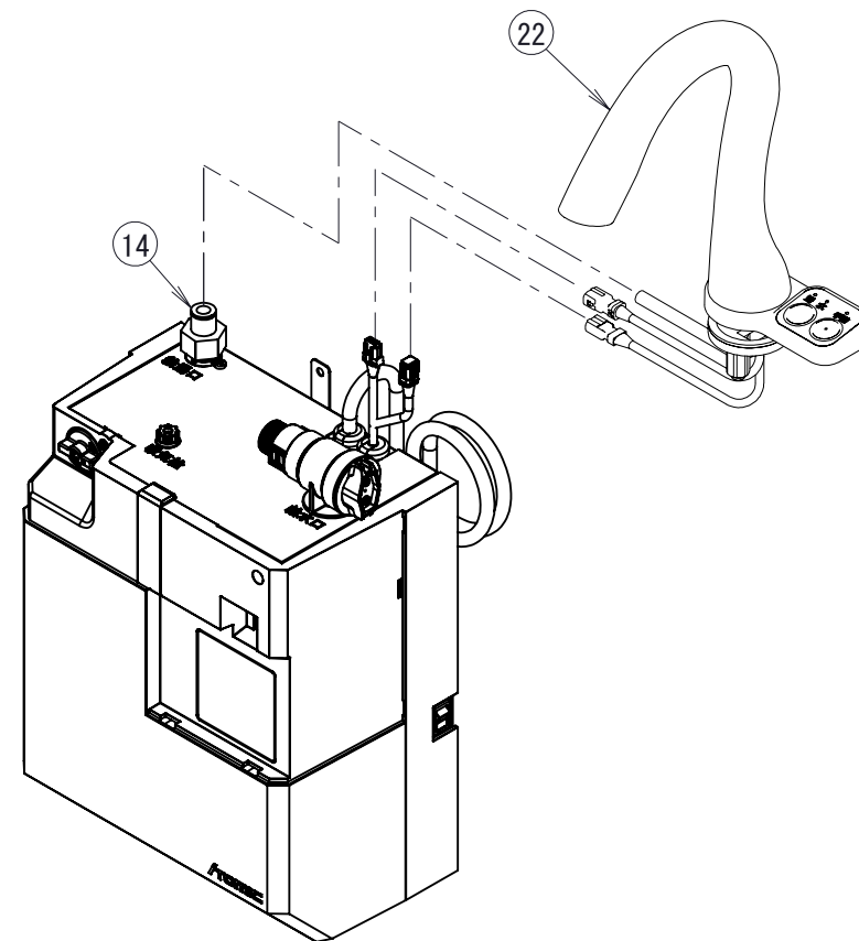
アイソメ図《自動水栓組立》
