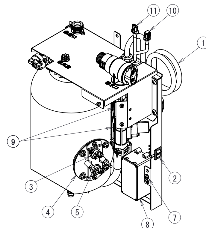
部品配置図 ESWM3AFW
