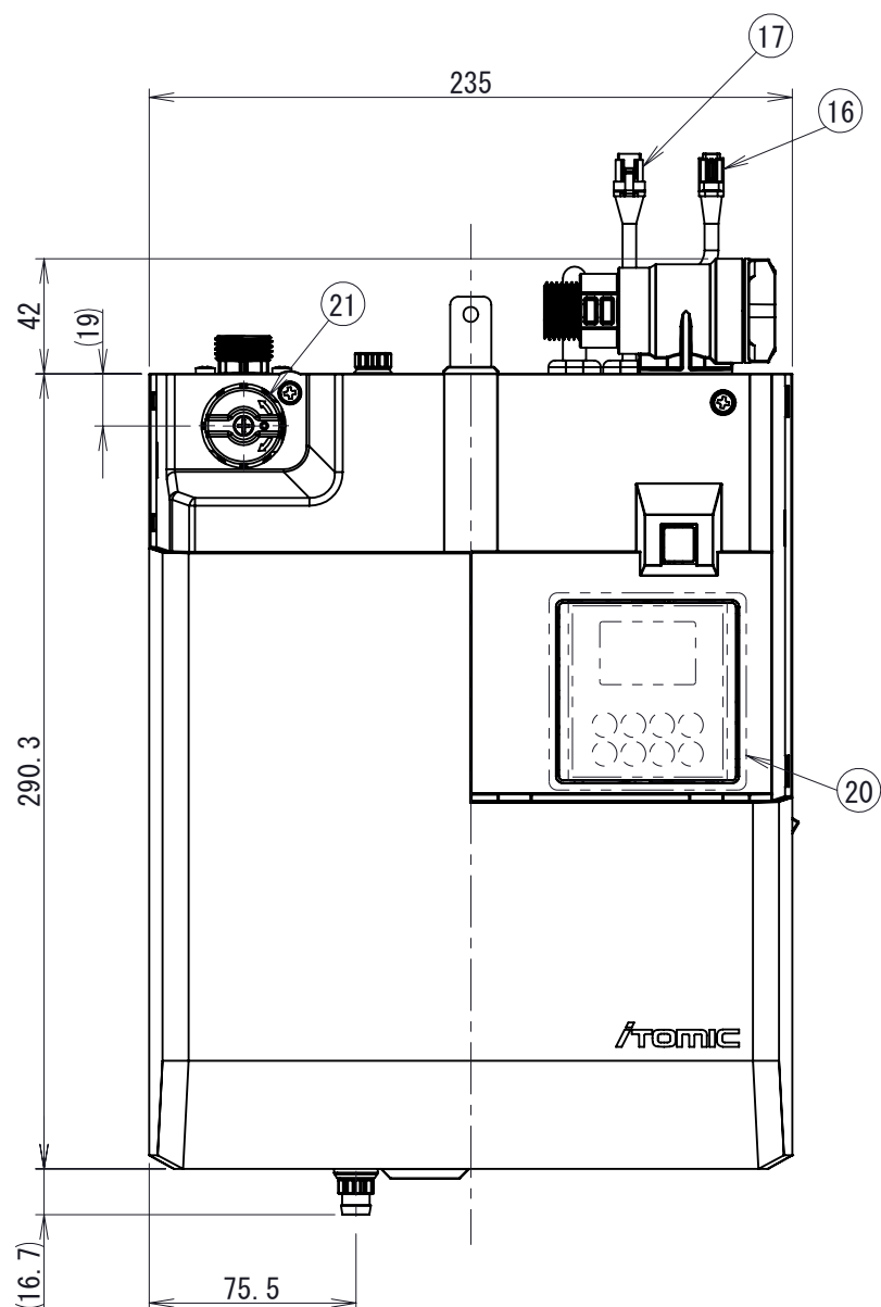
正面カバー取り外し状態詳細図
