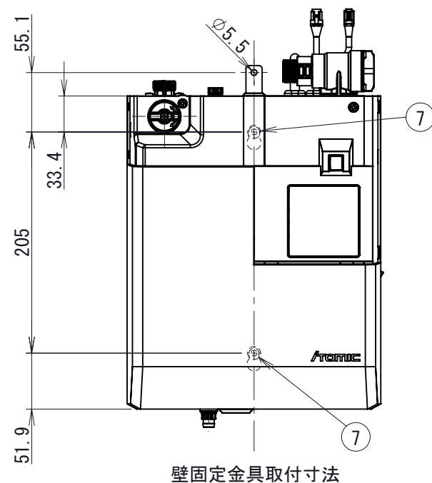
壁固定金具取付寸法
