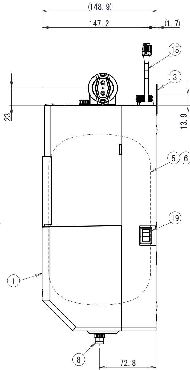
正面カバー取り外し状態詳細図
