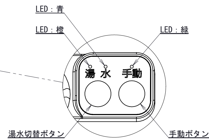
操作部詳細図
