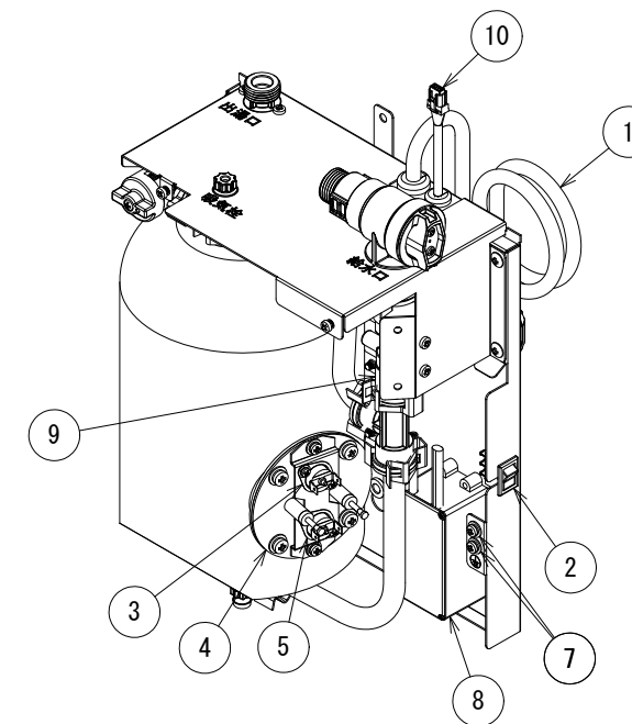
部品配置図 ESWM3ASW
