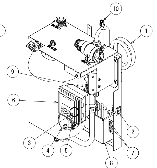
部品配置図 ESWM3TSW
